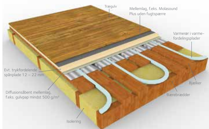
Eksempel på opbygning med bærebælter og varmefordelingsplader.
