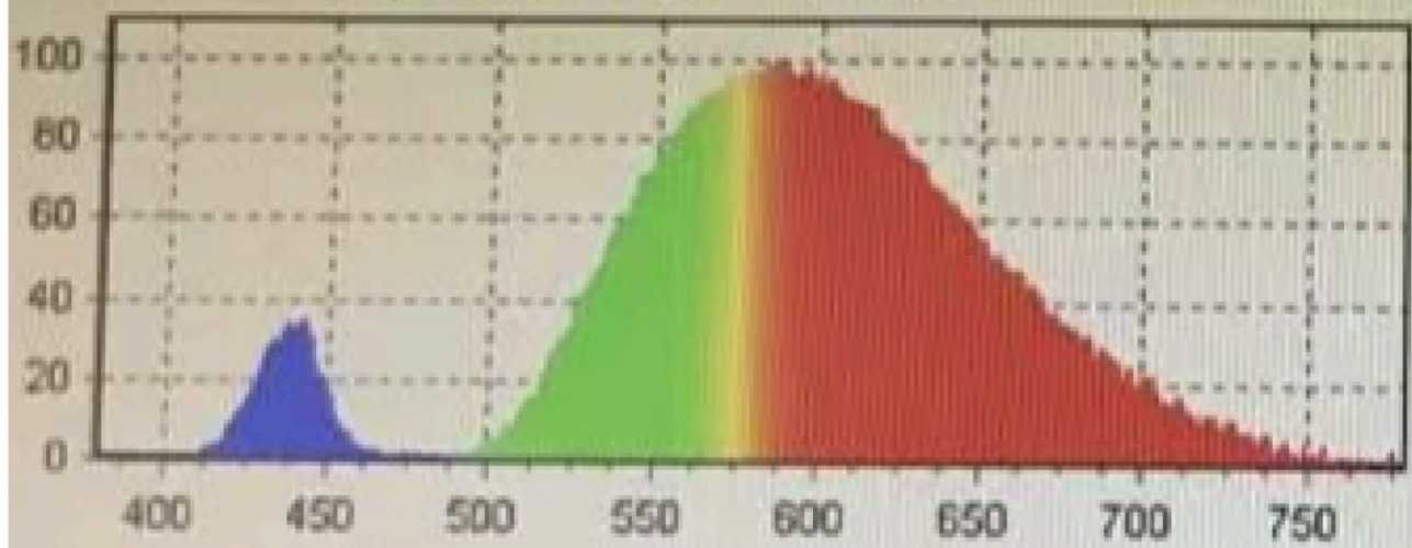
光谱相对能量百分比分布曲线
