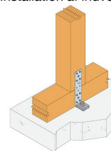
Fig. 3: Installation af indvendig væg
