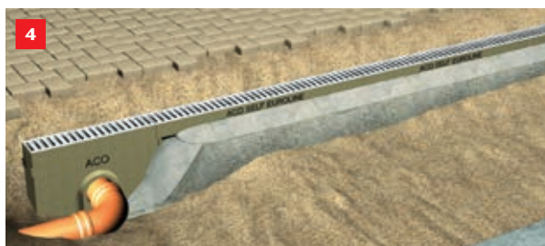
Betonen lægges op ad drænets sider, således at den første række fliser sættes i betonen. Det sikrer drænet mod side- værts bevægelser og tryk på drænets sidevægge.
