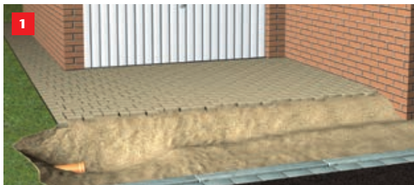
Fastlæg placering af linjedræn. Overvej belastningsklasse ifb. med kørsel på dræn. Grav en ca. 20-25 cm dyb rende til drænene.
