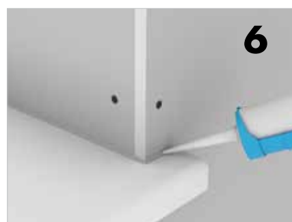
6. Efter montagen tættes med acrylfugemasse mellem elementet og de tilstødende flader.
