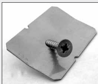
Fæsteskive (t= 1 mm) 36x55 mm, Skruer 5x35
